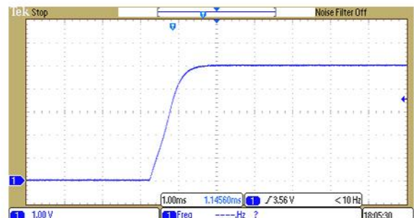
短路保护释放 VIN=25V, 短路保护释放
