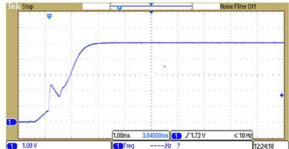
系统带载启动 带载30mA启动COUT=10uF
