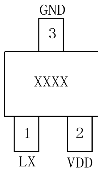
SOT23
