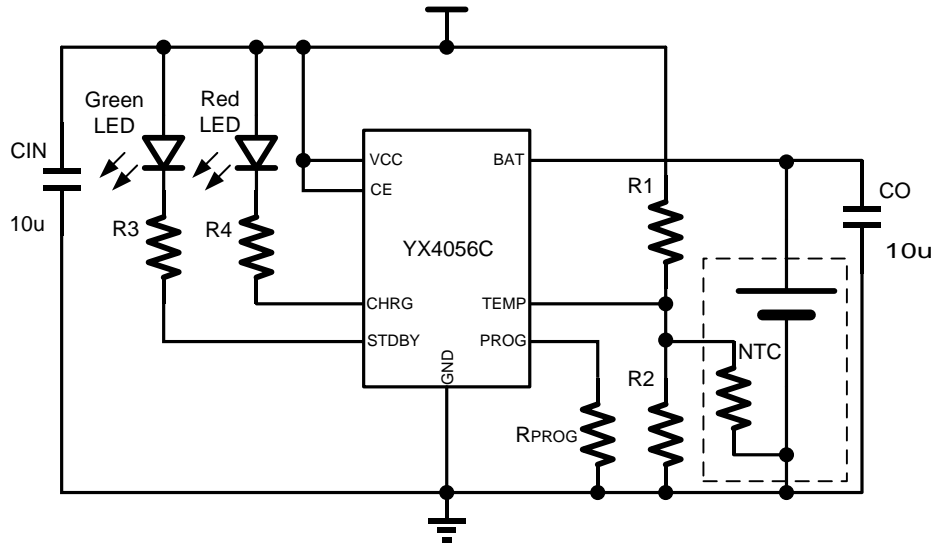
图 4. 典型应用电路
